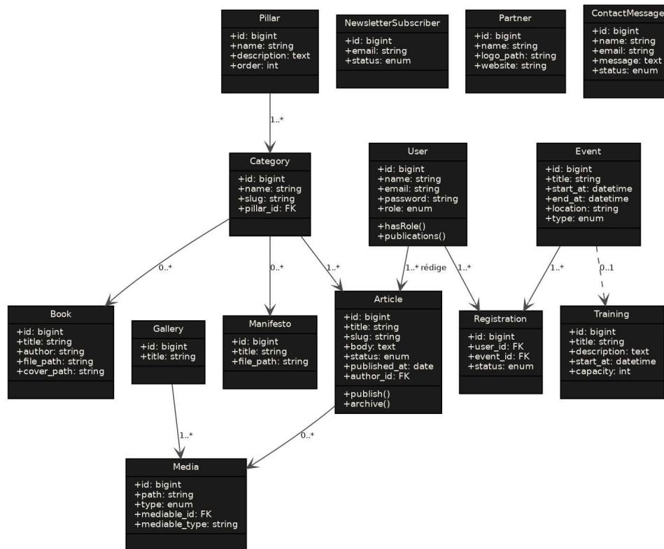
Figure 5 — Diagramme de classes (extrait des entités principales)
