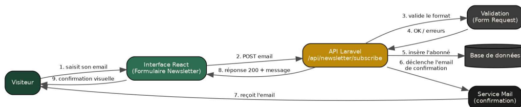
Figure 6 — Diagramme de séquence : inscription à la newsletter
