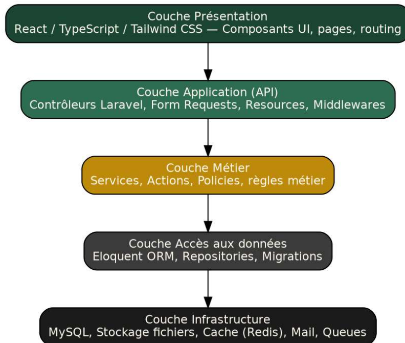
Figure 2 — Architecture logicielle en couches
