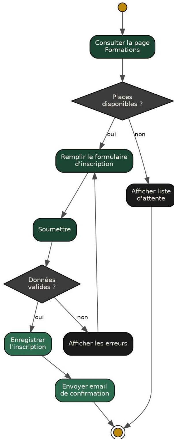
Figure 7 — Diagramme d'activité : inscription à une formation
