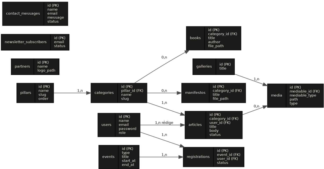
Figure 9 — Modèle conceptuel des données (extrait des entités principales)
